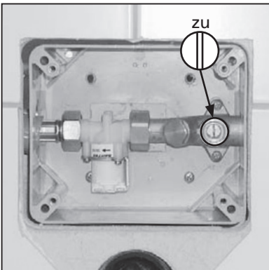
Vorabspernung schließen
