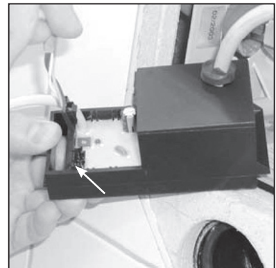
Sensorsiphon am Elektronikmodul anschließen. In umgekehrter Reihenfolge wieder zusammensetzen.
